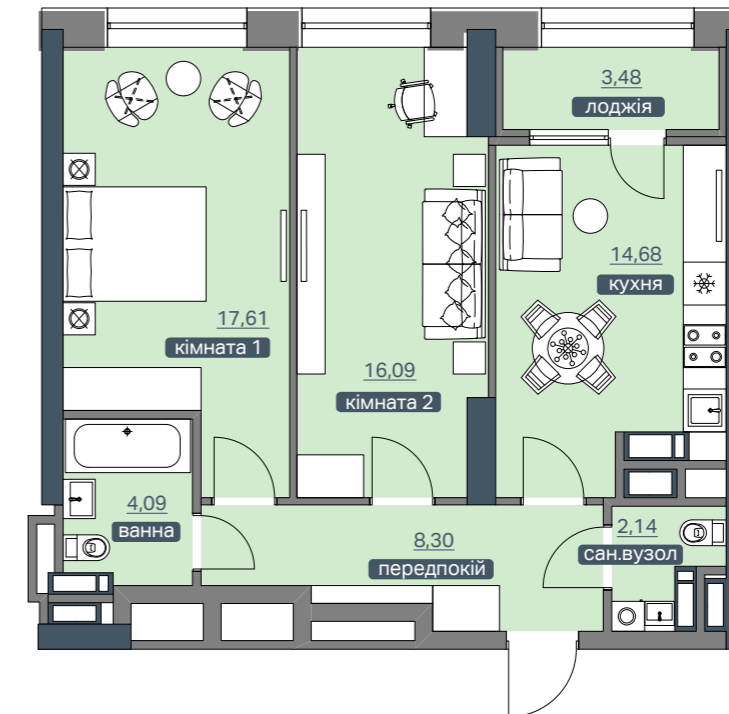
ПЛАН КВАРТИРИ
