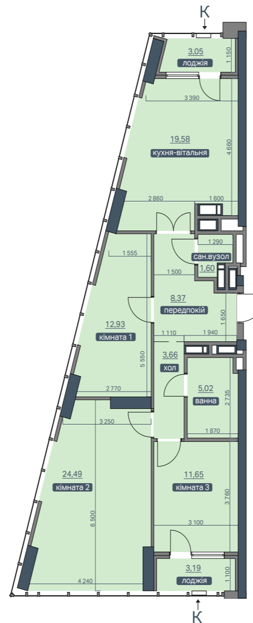
ПЛАН КВАРТИРИ З ОСНОВНИМИ РОЗМІРАМИ
