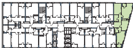
ПЛАН КВАРТИРИ
