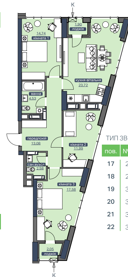
ПЛАН КВАРТИРИ
