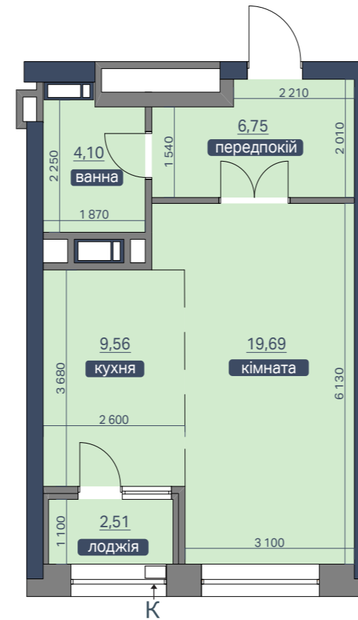
ПЛАН КВАРТИРИ З ОСНОВНИМИ РОЗМІРАМИ
