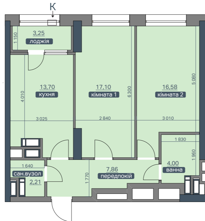
ПЛАН КВАРТИРИ З ОСНОВНИМИ РОЗМІРАМИ
