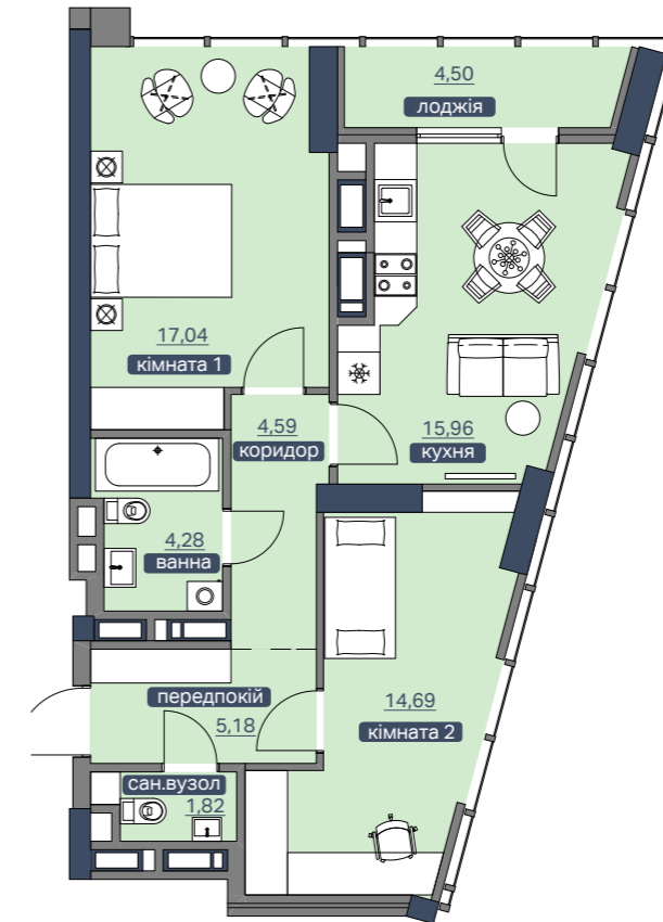
ПЛАН КВАРТИРИ
