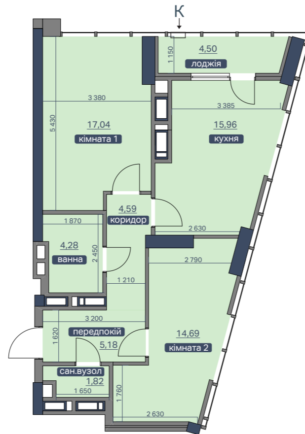
ПЛАН КВАРТИРИ З ОСНОВНИМИ РОЗМІРАМИ
