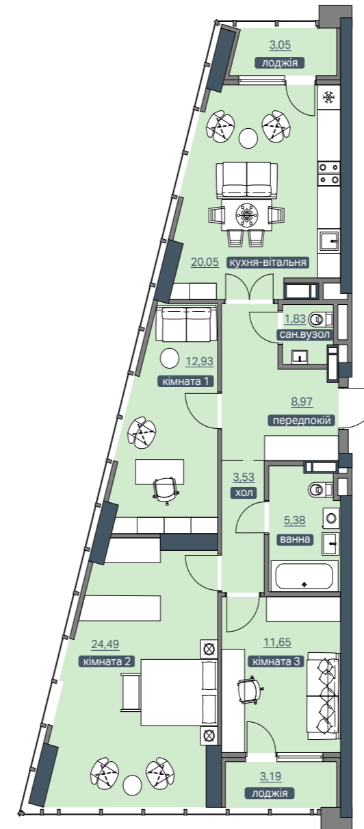
ПЛАН КВАРТИРИ
