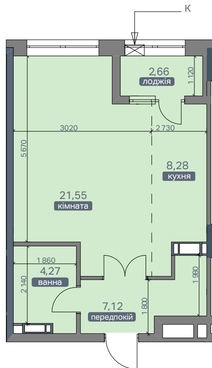
ПЛАН КВАРТИРИ З ОСНОВНИМИ РОЗМІРАМИ
