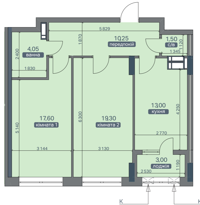
ПЛАН КВАРТИРИ З ОСНОВНИМИ РОЗМІРАМИ
