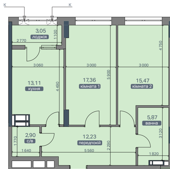
ПЛАН КВАРТИРИ З ОСНОВНИМИ РОЗМІРАМИ
