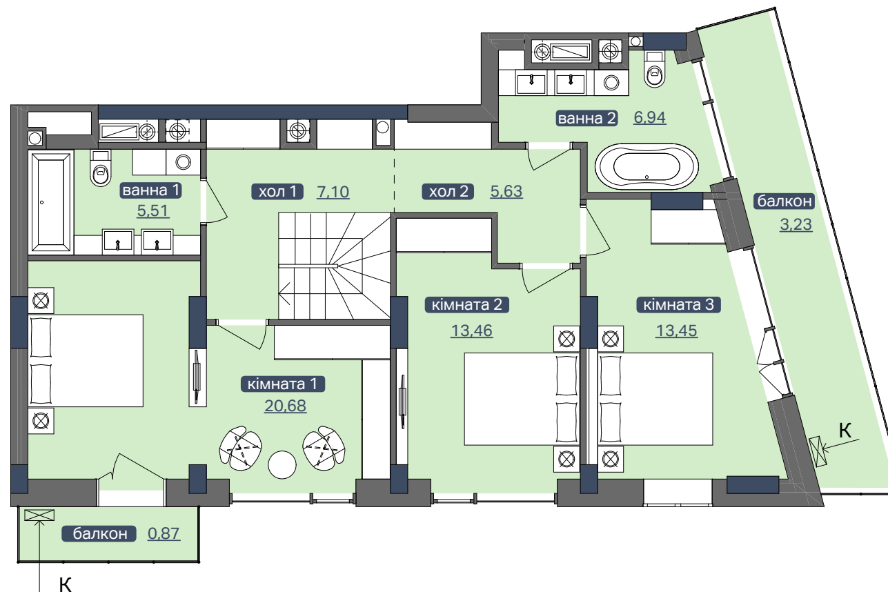
ПЛАН 10 ПОВЕРХУ
