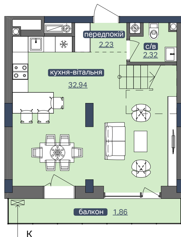
ПЛАН 9 ПОВЕРХУ
