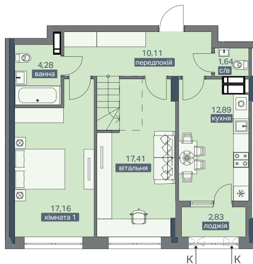
ПЛАН КВАРТИРИ - 9 ПОВЕРХ
