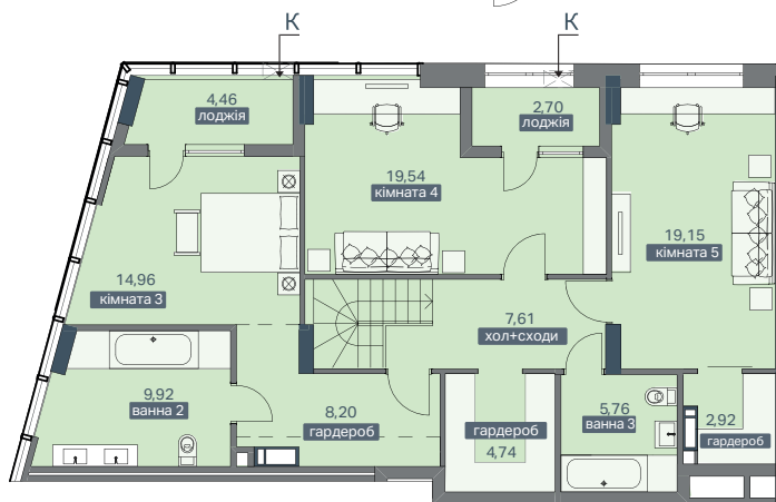
ПЛАН КВАРТИРИ 10 ПОВЕРХ
