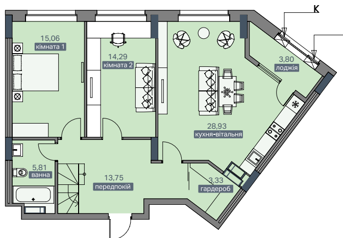
ПЛАН КВАРТИРИ 9 ПОВЕРХ
